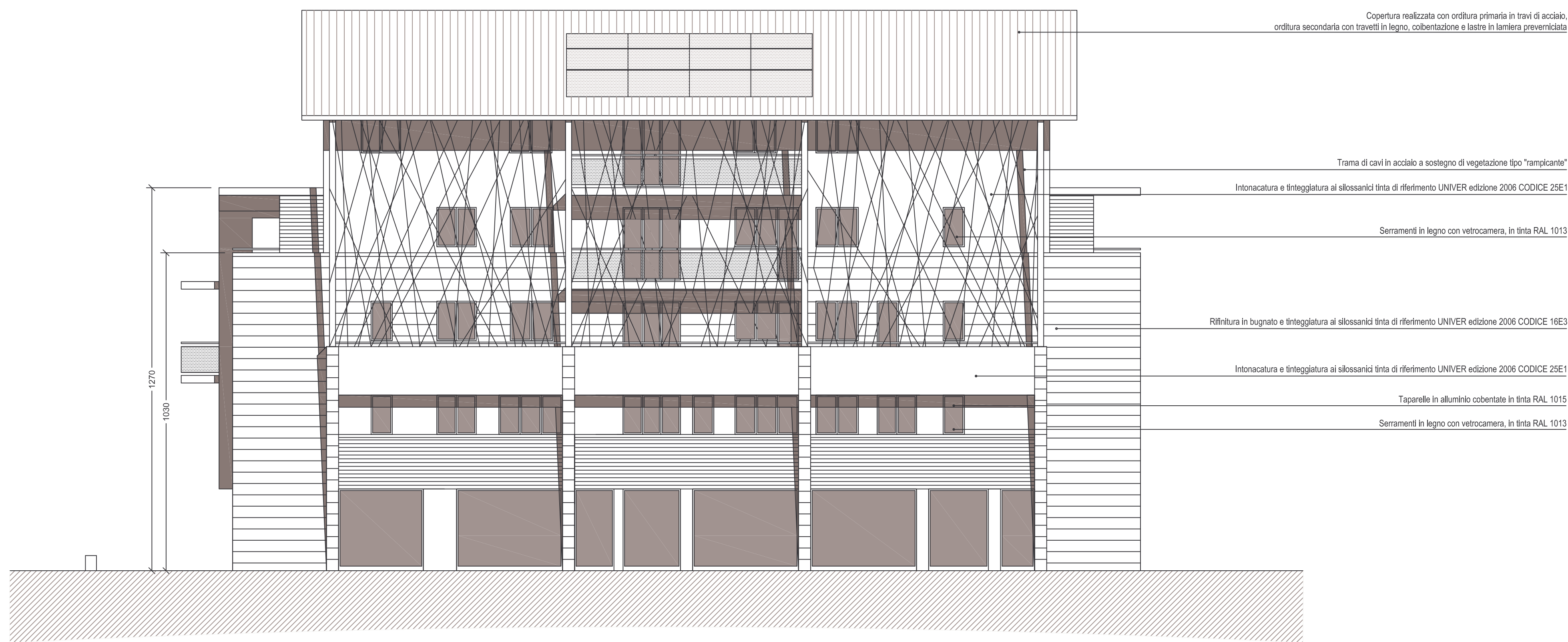
PROSPETTO SUD-EST
