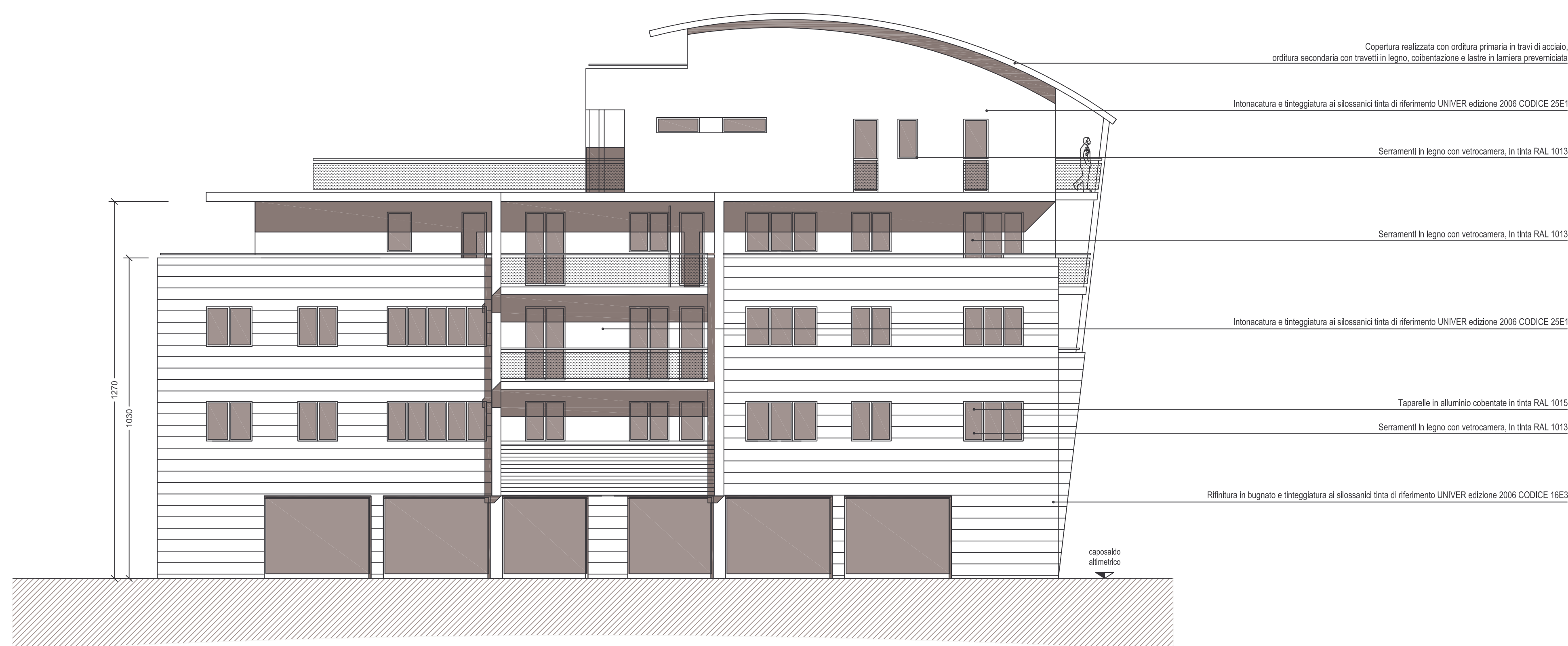
PROSPETTO SUD-OVEST
