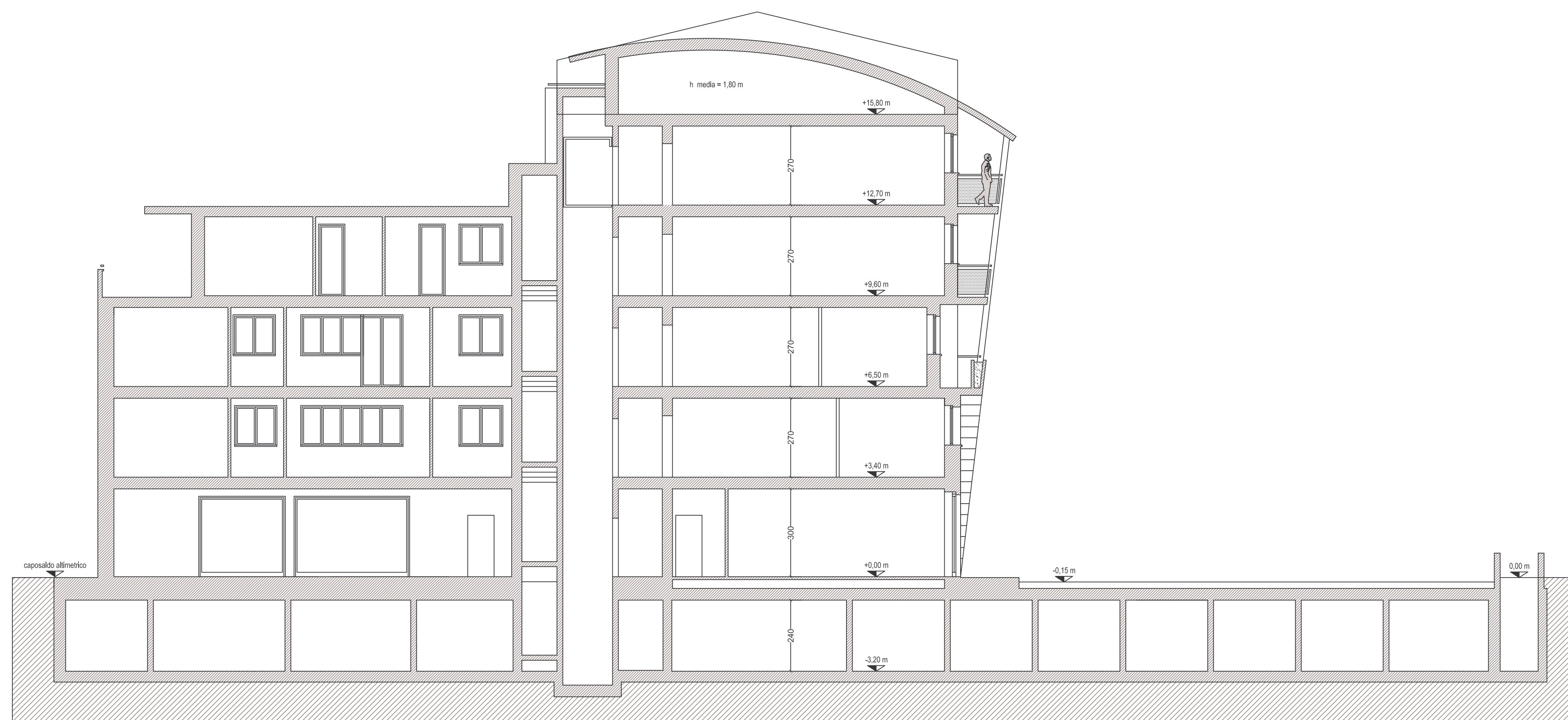
SEZIONE A-A
